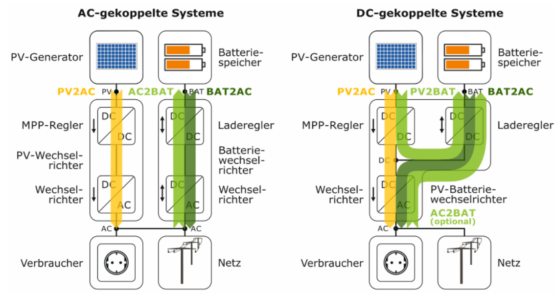
Abbildung 7 AC-/DC-Kopplung
